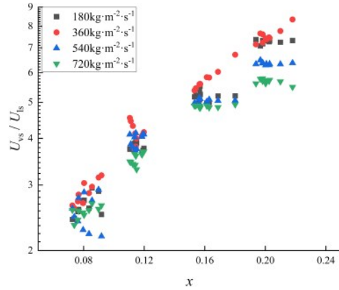
(c)不同质量流速下气液相速度比随干度的变化
