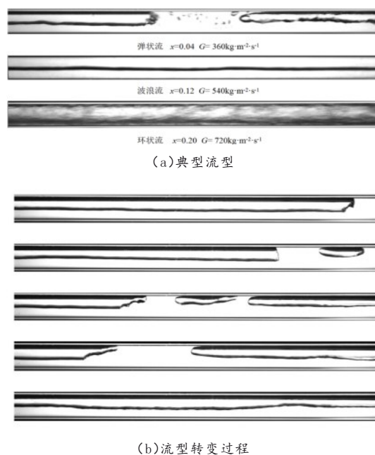
图4 实验典型流型及其转变过程
