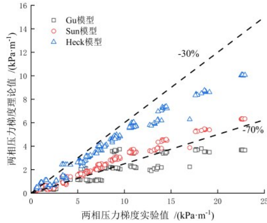
图 11 经典压降模型理论结果与实验数据的对比
