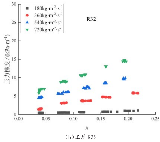
图9 不同工质摩擦压力梯度分布
