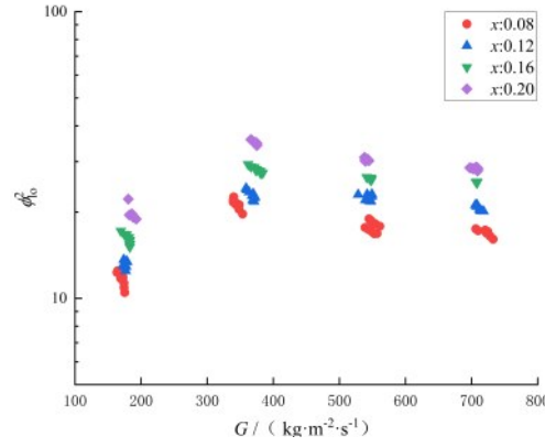
(b)不同干度下 \phi_{lo}^2 随质量流速的变化
