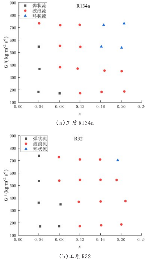
图5 不同工质流型的分布
