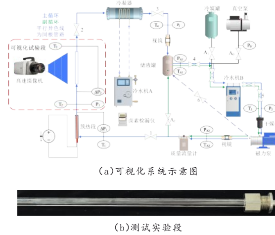
图 1 两相流动可视化试验系统示意图及测试试验段
