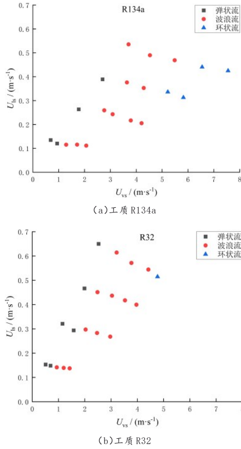
图6 不同工质液气相表观速度 U_{ls} 和 U_{vs} 的对比
