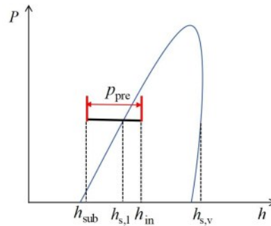
图 2 工质预热过程压焓图
