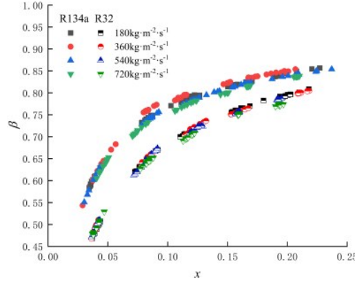
图8 不同质量流速下两种工质截面含气率随干度的变化
