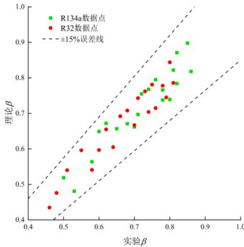
图7 截面含气率误差分析
