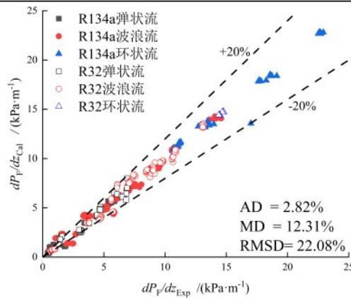
图12 本文所构建模型的预测结果分析
