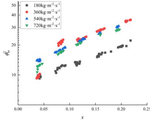
(a)不同质量流速下 \phi_{lo}^2 随干度的变化
